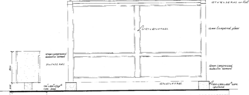
ELEVATION 3
